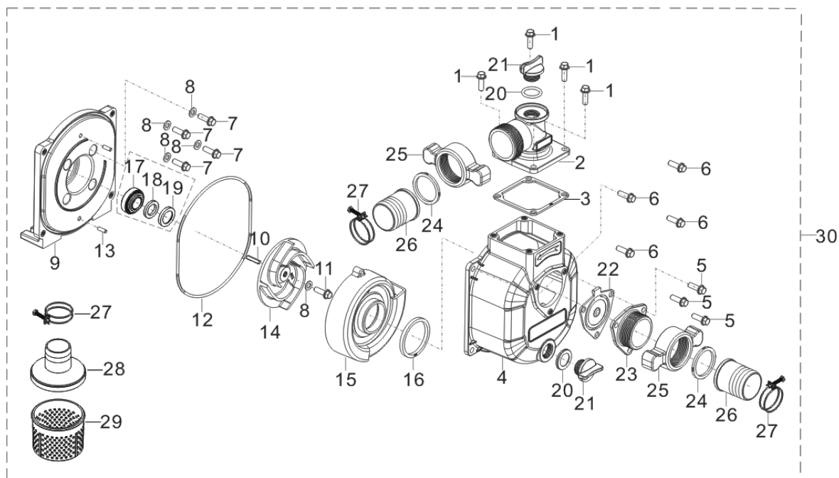
FIG.15 (E15 )
