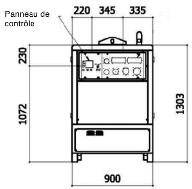
VUE AVANT
